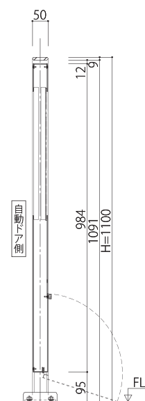
【断面図】
